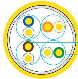
US-9488LSZH : CAT 8 S/FTP CABLE, LSZH
